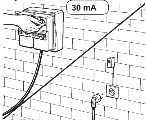
Collegamento elettrico.
