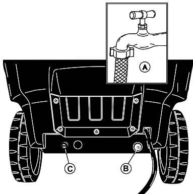
Conexión hídrica.
